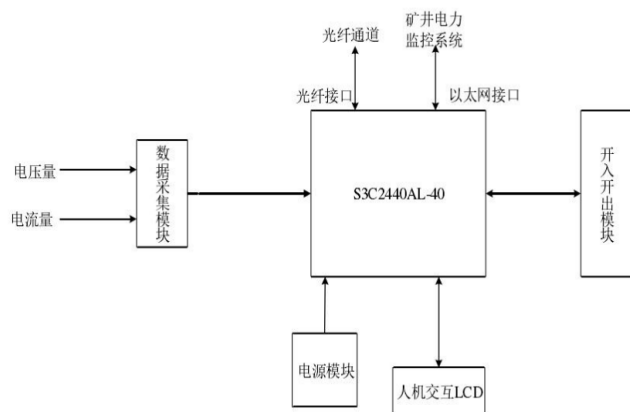
图2 防越级跳闸保护装置结构图
