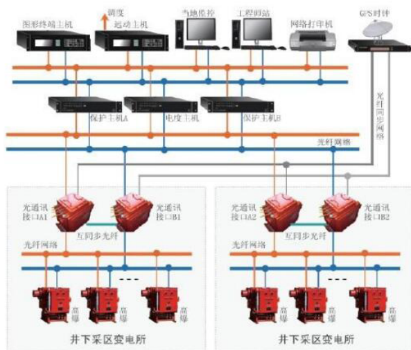
图1 防越级跳闸保护系统框架图
