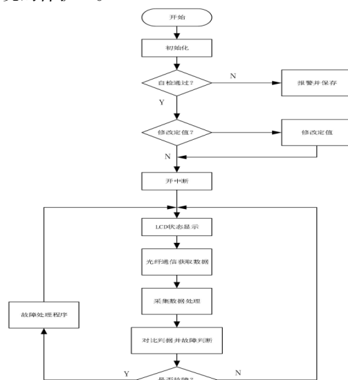
图3 故障处理流程示意图
