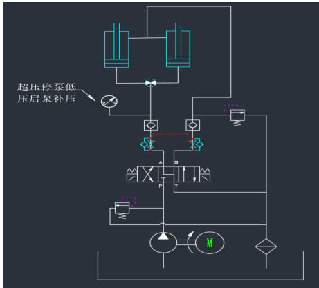
图 3 液压控制
