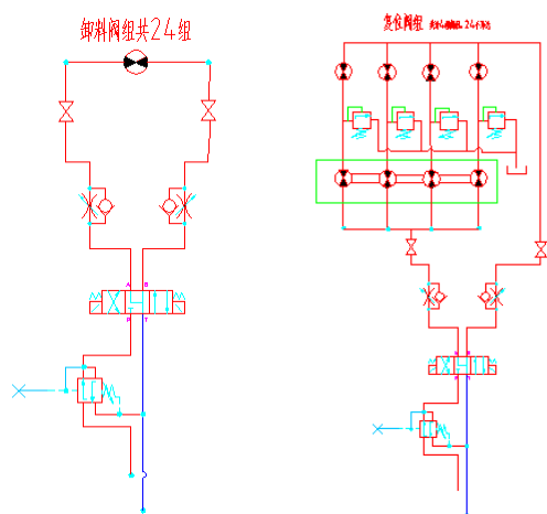
图1 改造后液压原理图 (此阀组共24组)
